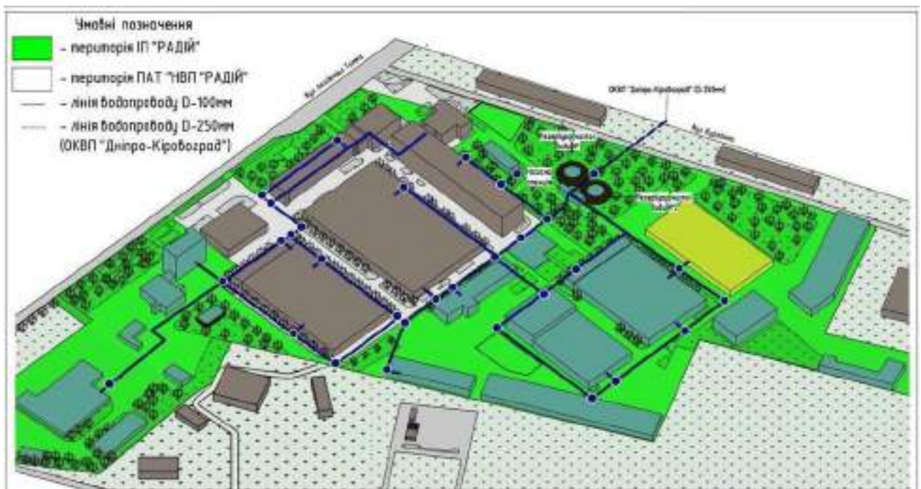
Мал. 5. Схема розташування мереж і об'єктів системи водопостачання
