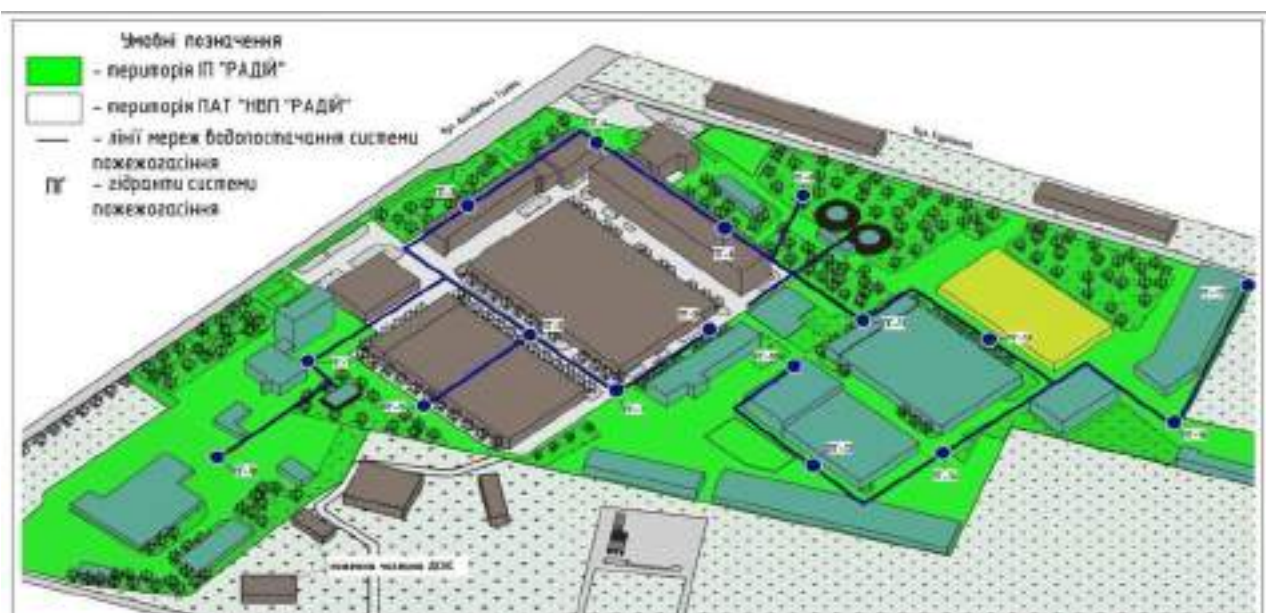
Мал.8 Схема розташування мереж та об'єктів системи пожежогасіння
